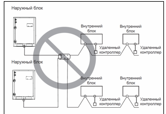
Многожильный кабель
