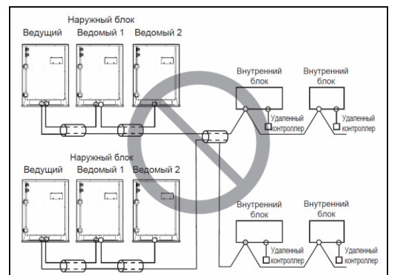
Многожильный кабель
